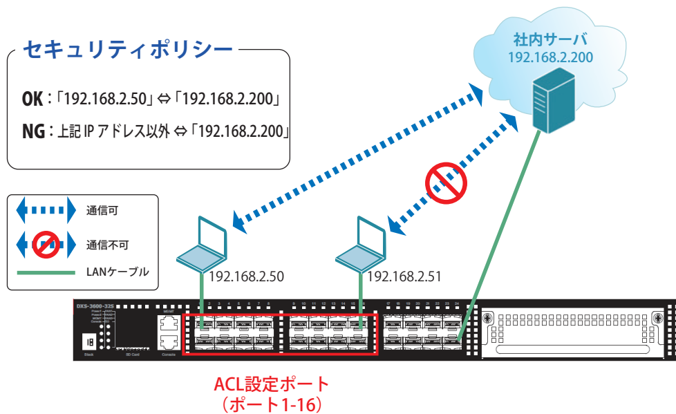
図 76-4 Access List (DXS-3600-32S)
