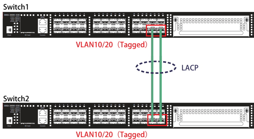
図 76-3 Link Aggregation (DXS-3600-32S)
