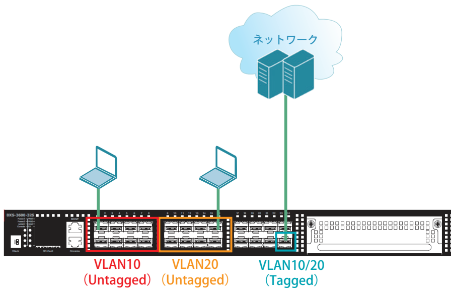
図 76-2 VLAN (DXS-3600-32S)
