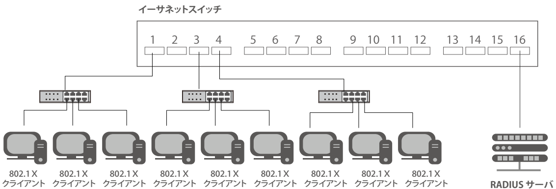
図 12-8 ホストベースアクセスコントロールのネットワーク構成例
