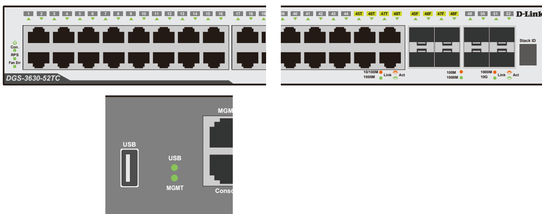
図 3-10 DGS-3630-52TC の背面パネル LED 配置図 (上: 前面 / 下: 背面)
