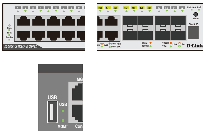
図 3-11 DGS-3630-52PC の背面パネル LED 配置図 (上: 前面 / 下: 背面)
