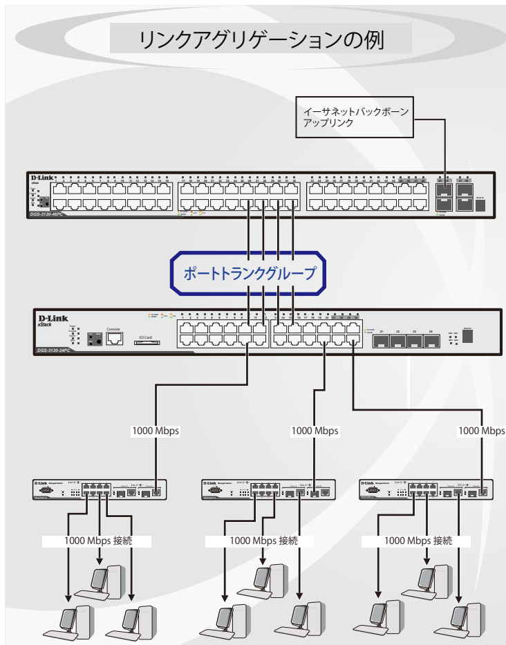
図 8-63 ポートトランクグループの例
