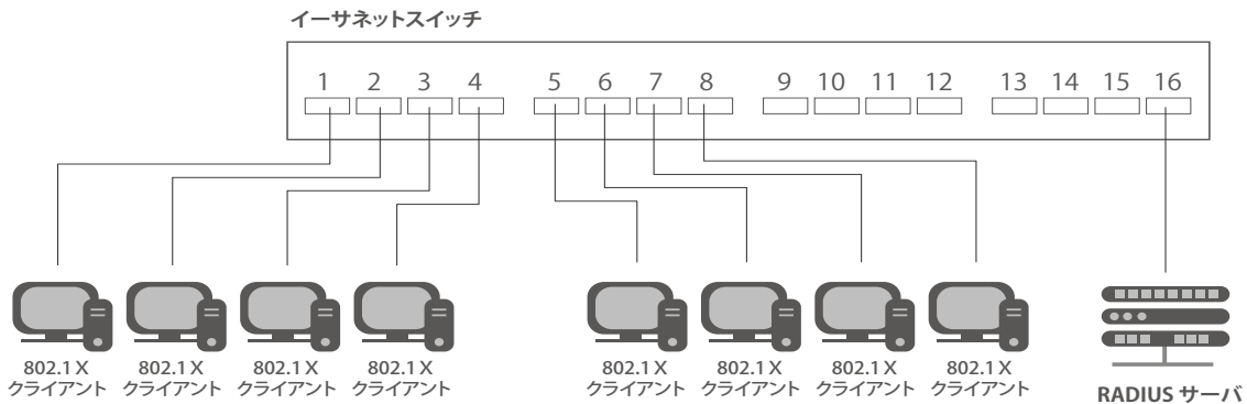
図 12-7 ポートベースアクセスコントロールのネットワーク構成例
