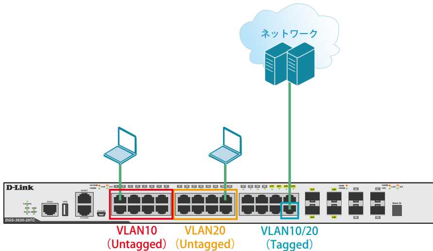
図 20-2 VLAN (DGS-3630-28TC)
