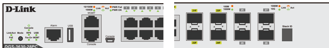
図 3-9 DGS-3630-28PC の前面パネル LED 配置図
