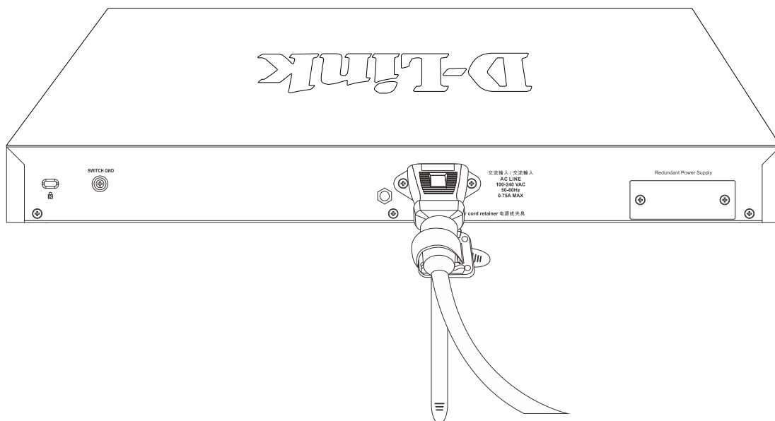
図 2-9 電源抜け防止器具の固定確認
