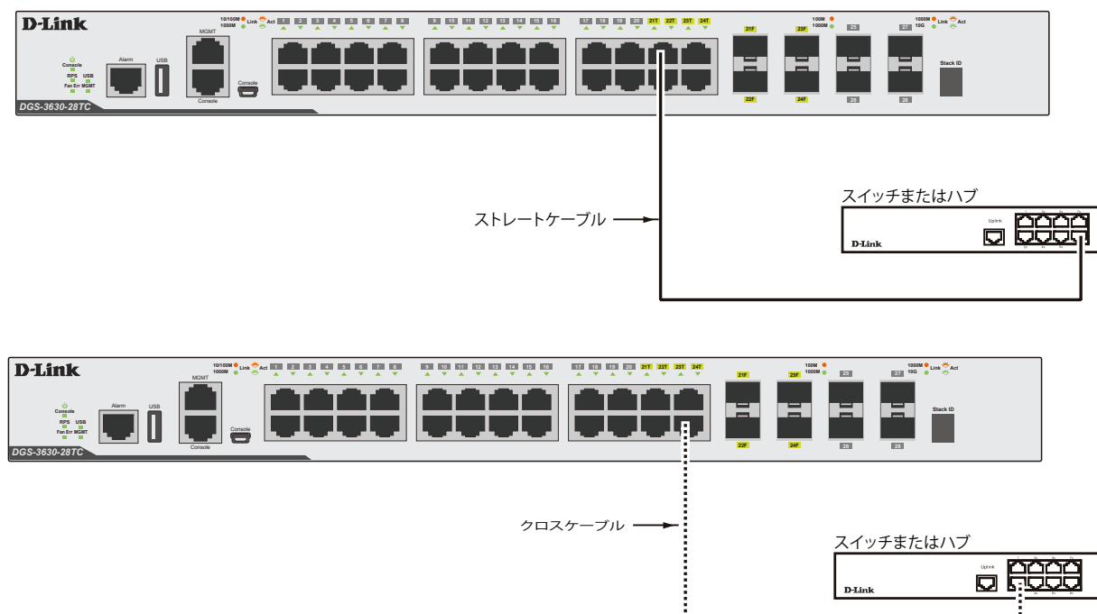
図 3-2 ストレート、クロスケーブルでハブまたはスイッチと接続する図
