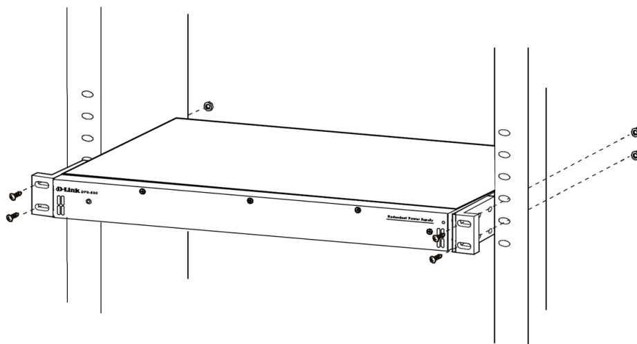
図 2-11 DPS-700 をラックに取り付ける
