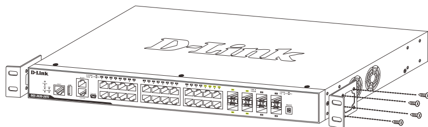
図 2-2 スイッチへのブラケットの取り付け図
