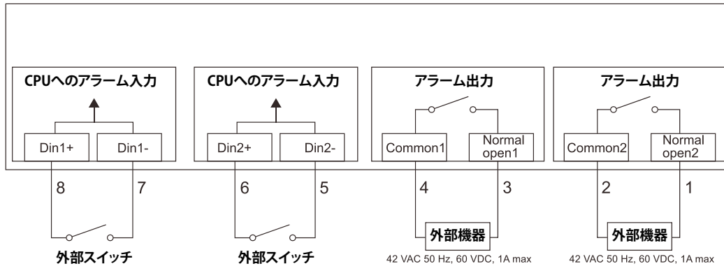
図 3-6 アラームコネクタ
