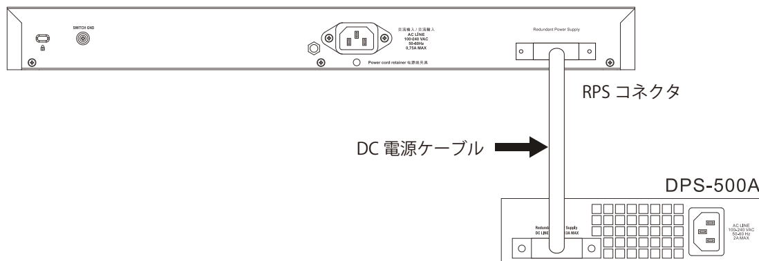
図 2-10 DGS-3630-28TC/SC と DPS-500A RPS の接続
