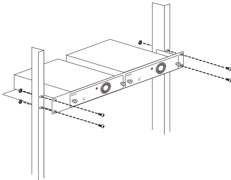
図 2-14 DPS-800 をラックに取り付ける
