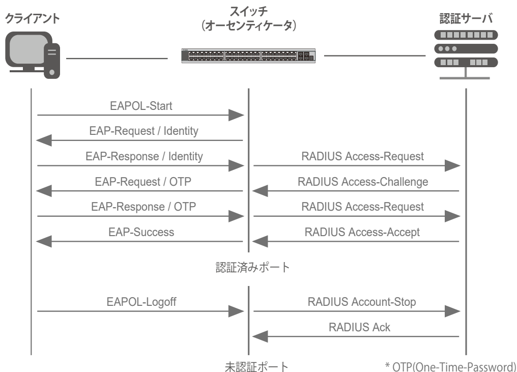
図 12-6 802.1X 認証プロセス
