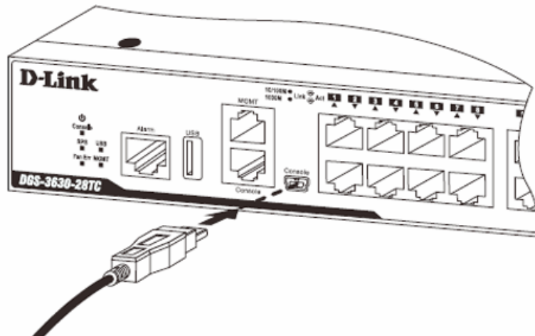
図 4-4 Mini-USB コンソールポートの接続
