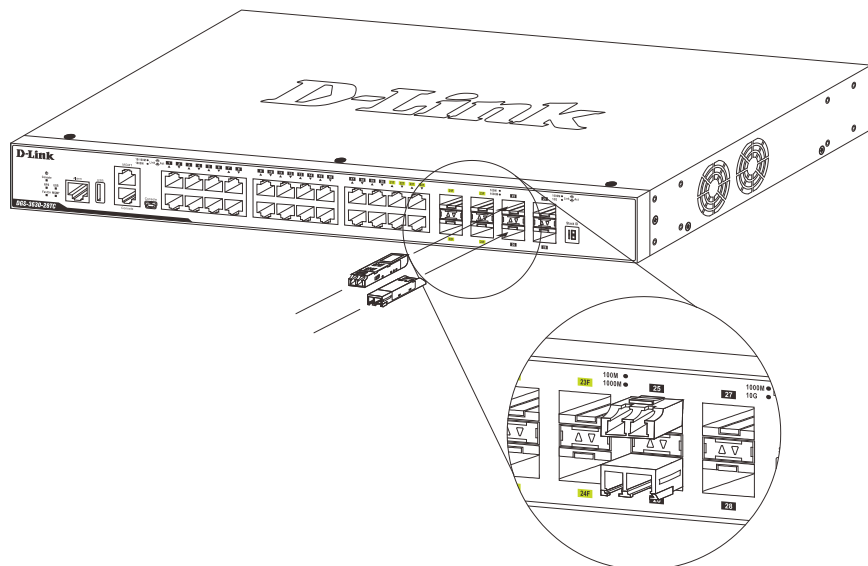
図 2-4 DGS-3630 シリーズ前面パネルの SFP ポートへのモジュールの挿入
