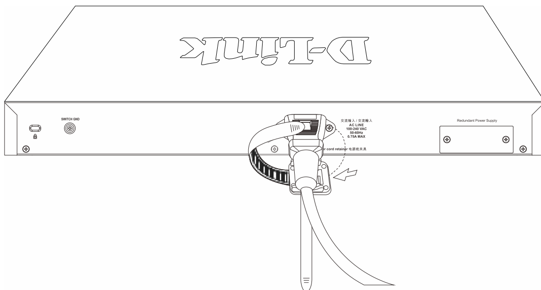
図 2-8 リテイナーの巻き付け、固定
