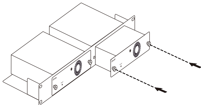
図 2-13 DPS-500A を DPS-800 に取り付ける
