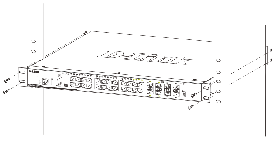
図 2-3 スイッチのラックへの設置図
