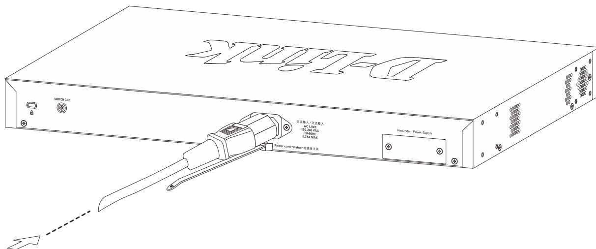
図 2-6 電源コード挿し込み
