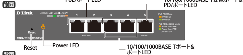
DGS-1100-05PDV2 10/100/1000BASE-T PoE給電ポート&PoE/ポートLED
