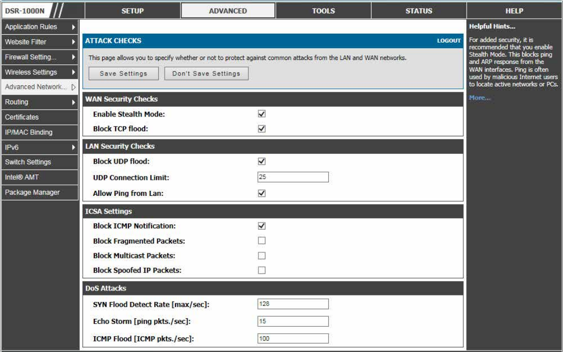
図 7-36 インターネット攻撃からルータと LAN を保護する
