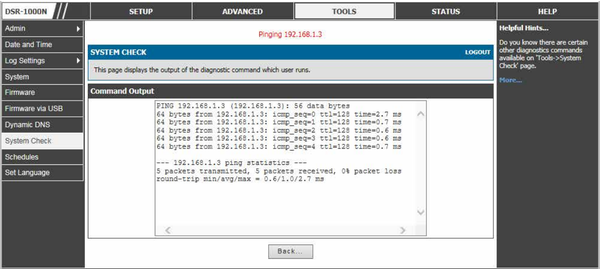
図 11-21 GUI で利用可能なルータ診断ツール - Ping
