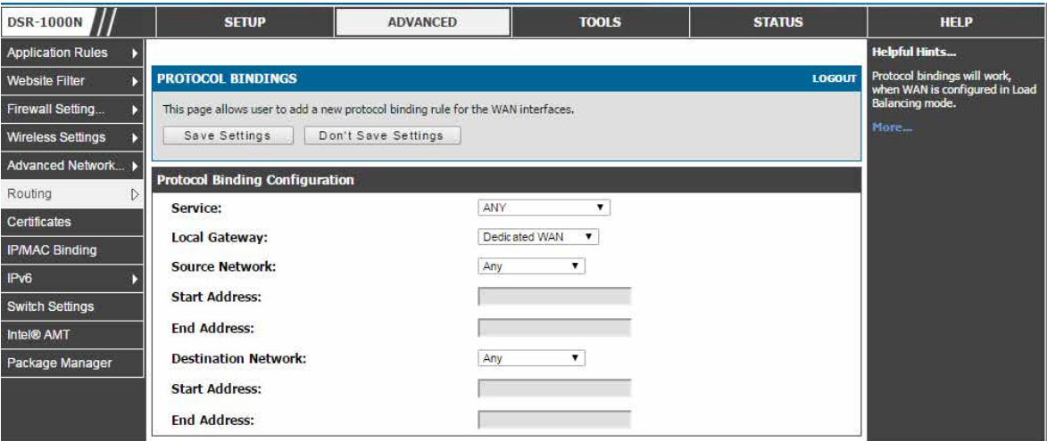
図 5-28 PROTOCOL BINDINGS 画面 - 追加
