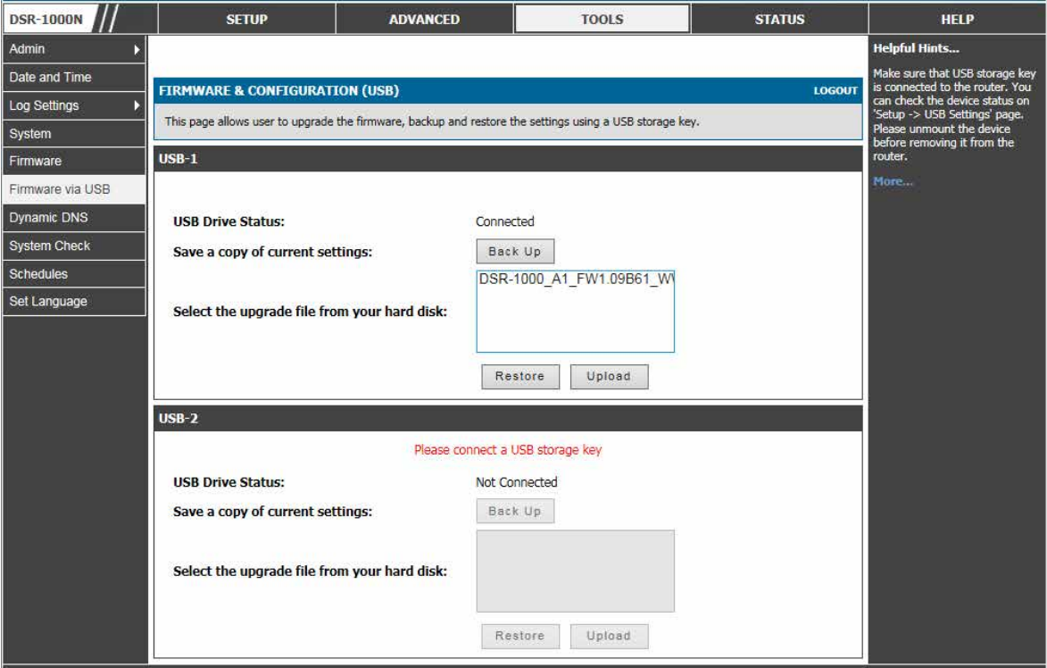
図 11-18 USB を使用したファームウェアバージョンとアップグレードオプション
