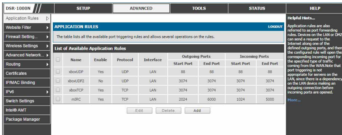
図 7-24 4 個のユニークなルールを表示する利用可能なアプリケーションルールのリスト
