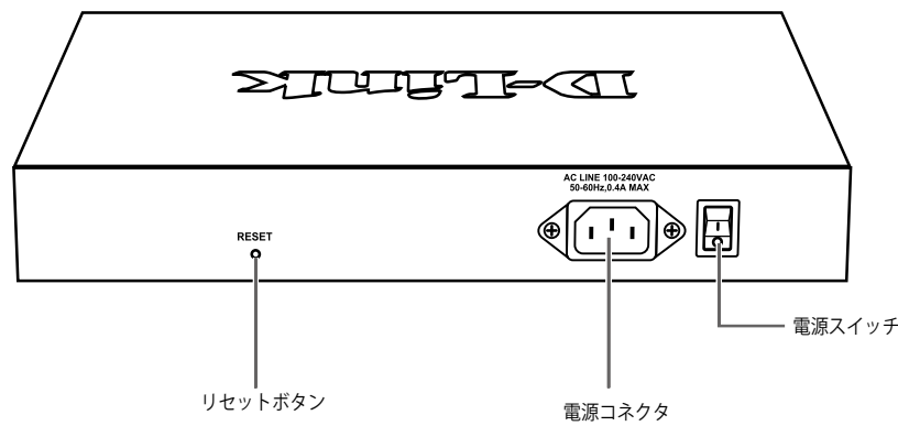
図 1-5 背面パネル図
