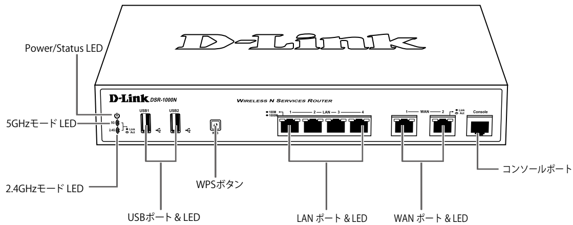
図 1-3 前面パネル図
