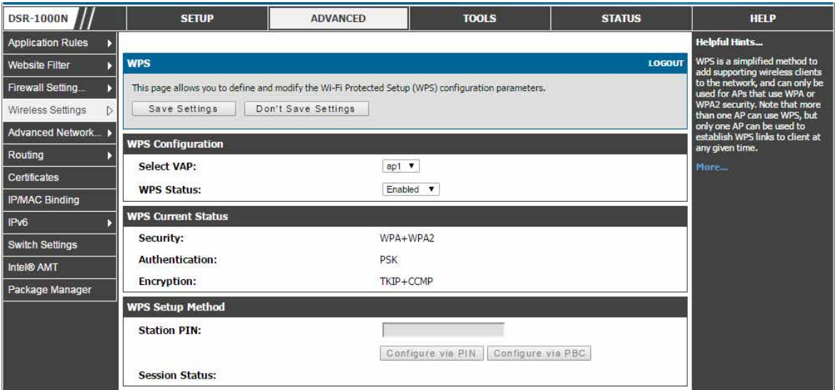
図 6-20 WPA/WPA2 プロファイルを持つ AP の WPS 設定
