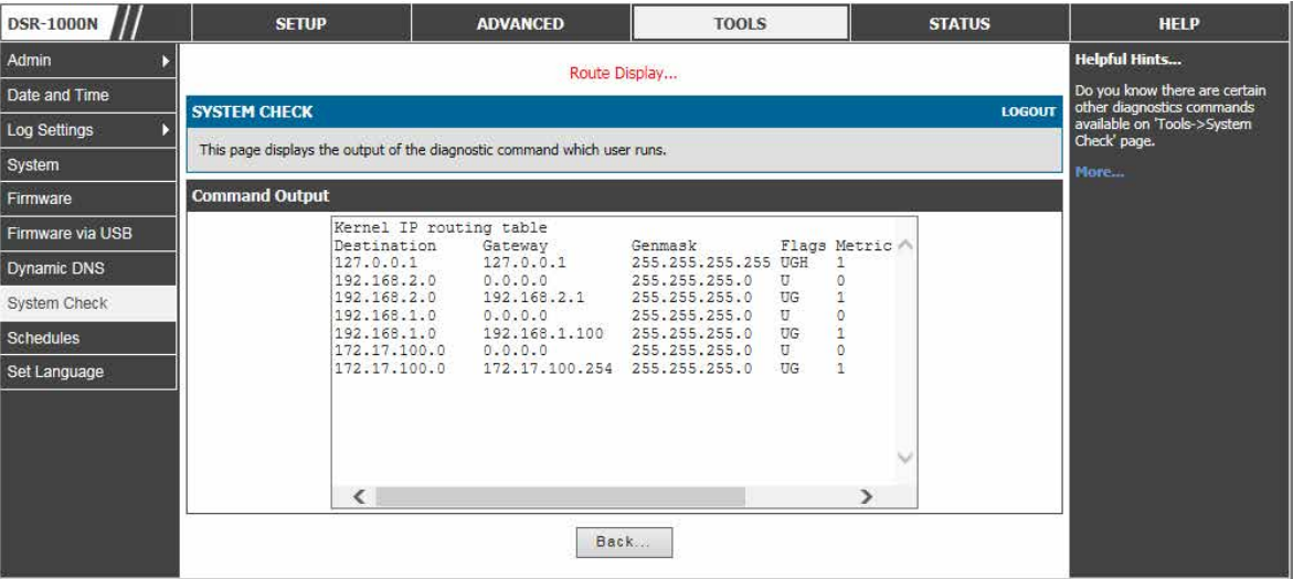
図 11-24 ルーティングテーブル出力
