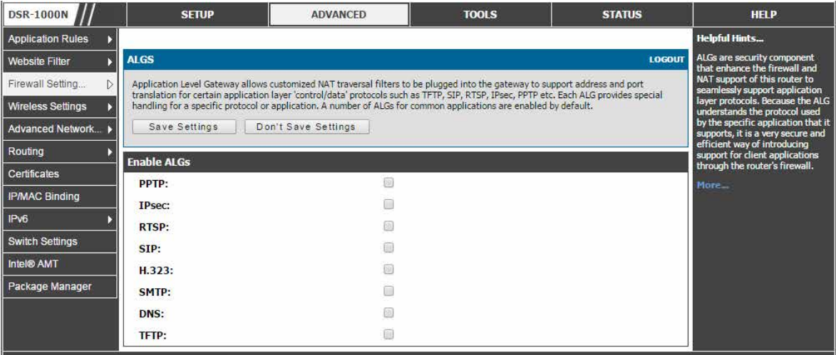
図 7-13 ルータにおける利用可能な ALG のでサポート
