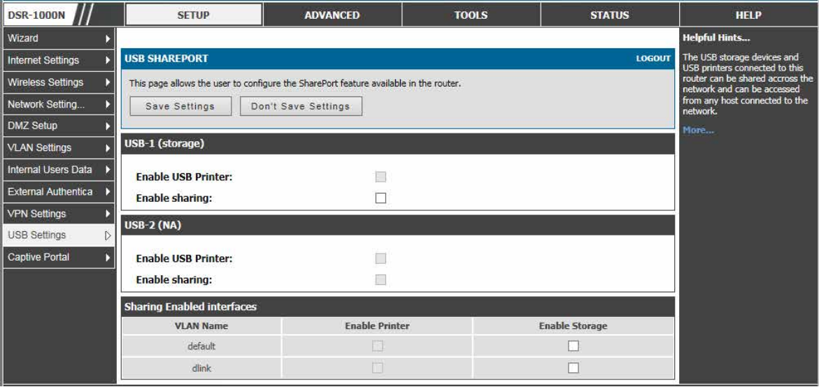
図 10-26 USB 共有ポートの設定
