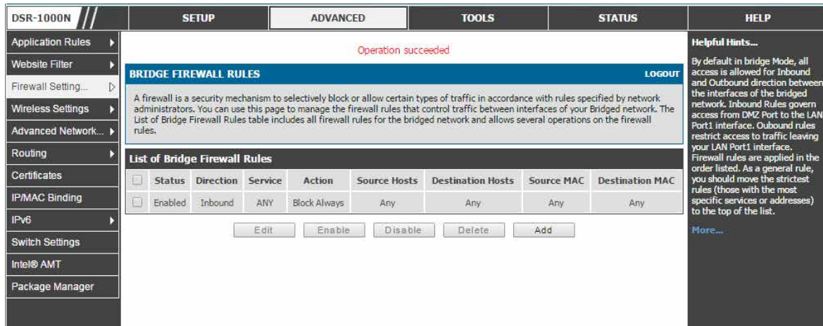
図 7-22 ブリッジファイアウォールルールのリスト
