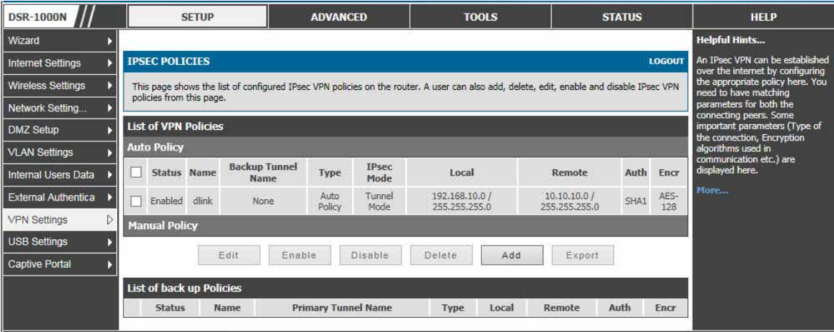
図 8-7 IPSec ポリシーリスト画面
