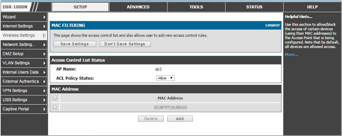
図 6-13 アクセスコントロールリスト表示画面
