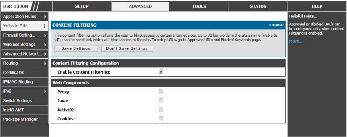
図 7-27 コンテンツフィルタリング設定
