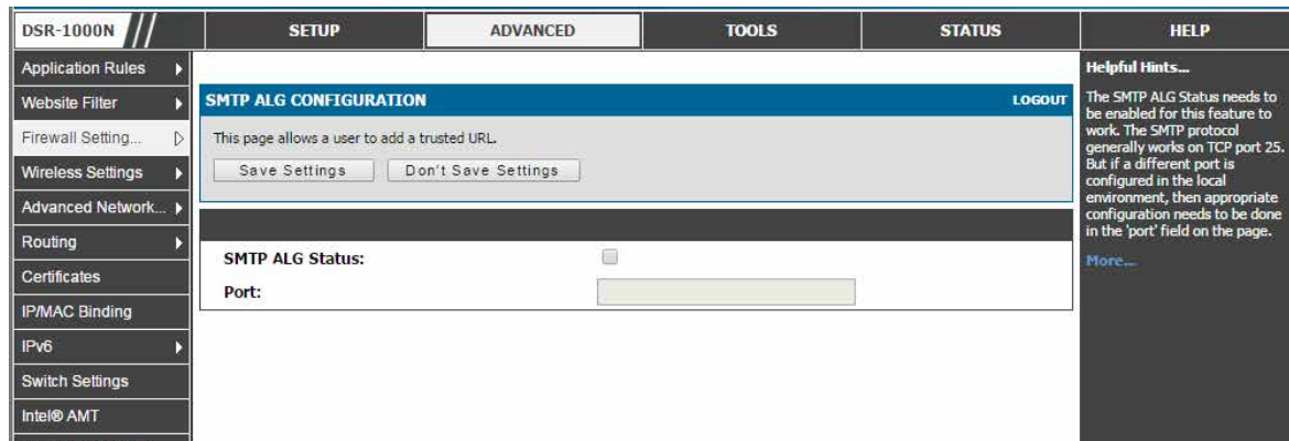
図 7-14 SMTP ALG 設定
