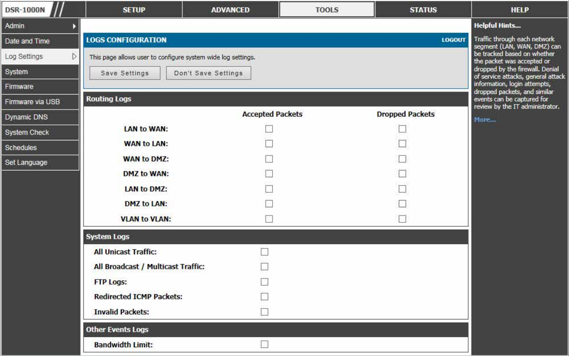
図 11-10 ルータを経由するトラフィックのためのログ設定オプション
