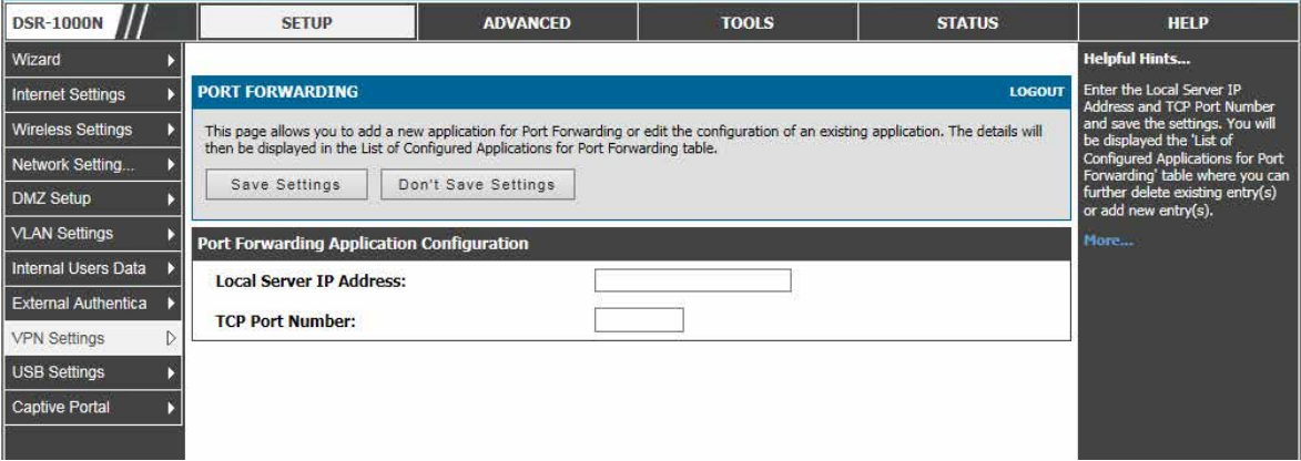
図 9-18 アプリケーションの設定画面
