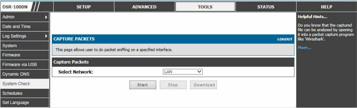
図 11-25 パケットキャプチャ
