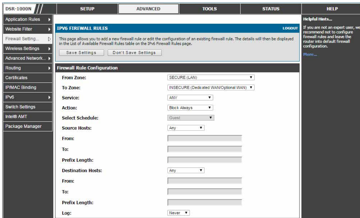
図 7-9 IPv6 ファイアウォールルール追加画面
