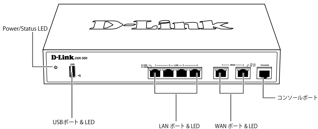
図 1-1 前面パネル図 (DSR-500)
