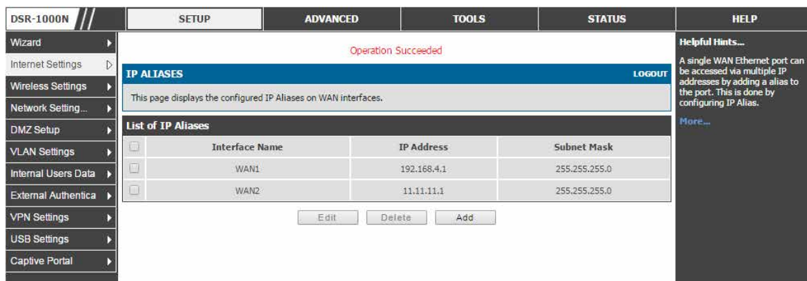
図 5-29 IP ALIASES 画面
