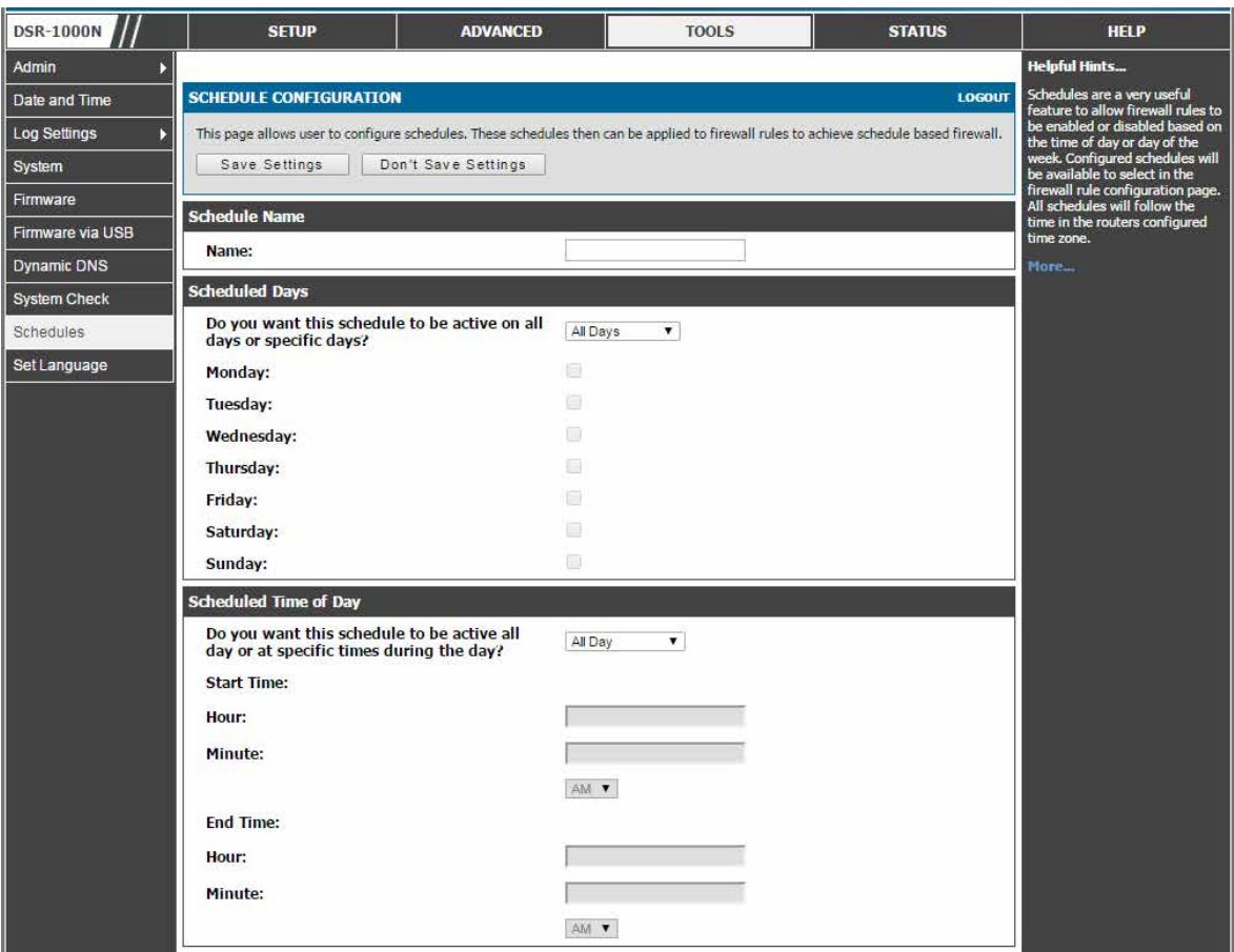
図 7-4 SCHEDULE CONFIGURATION 画面 - 追加
