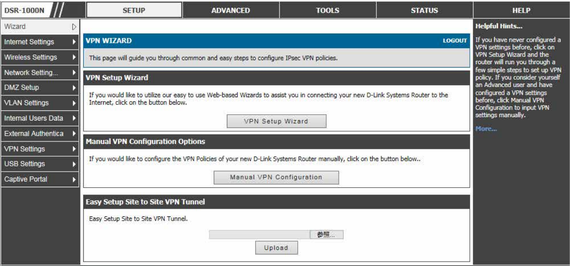
図 8-3 VPN ウィザードの開始画面
