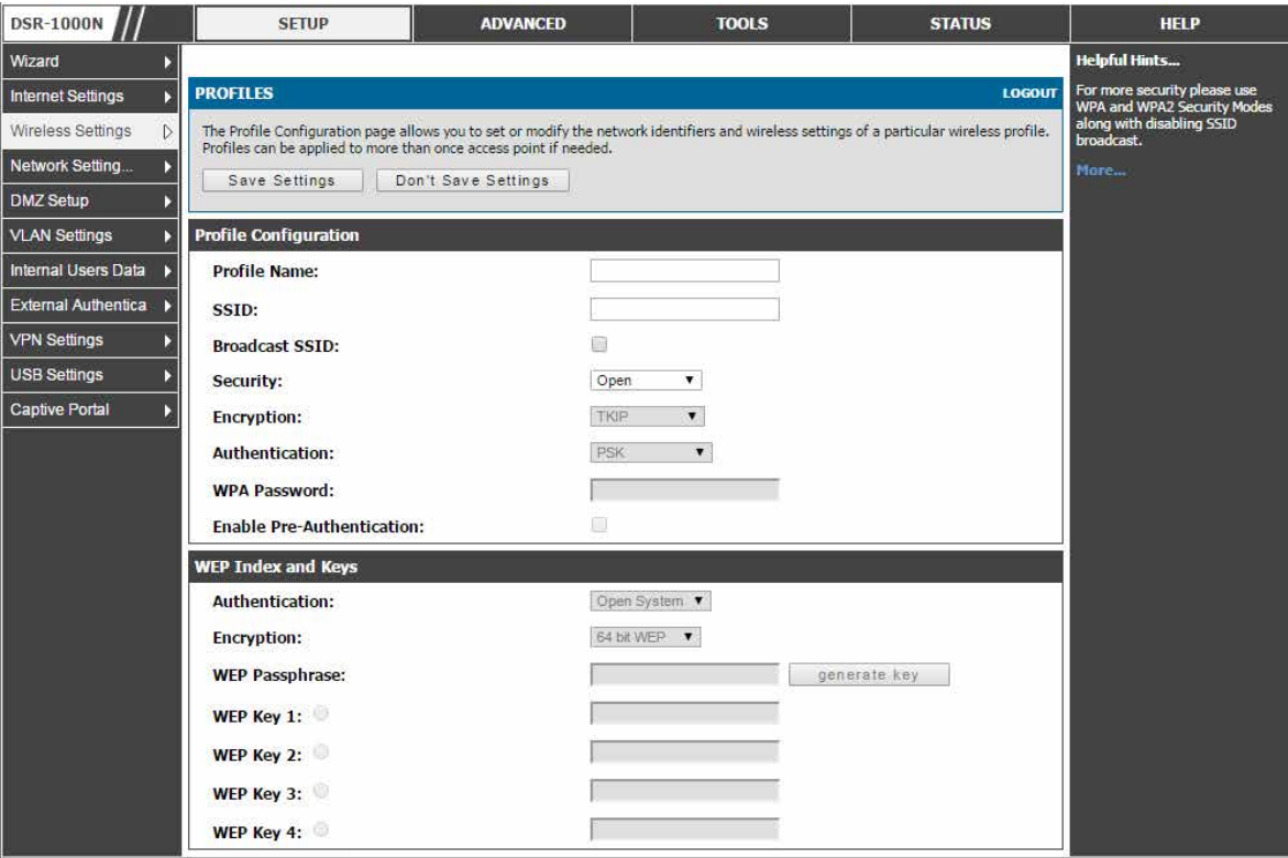
図 6-8 PROFILES 画面 - Add
