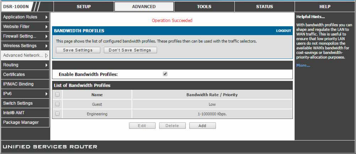
図 5-17 設定済み帯域幅プロファイルのリスト
