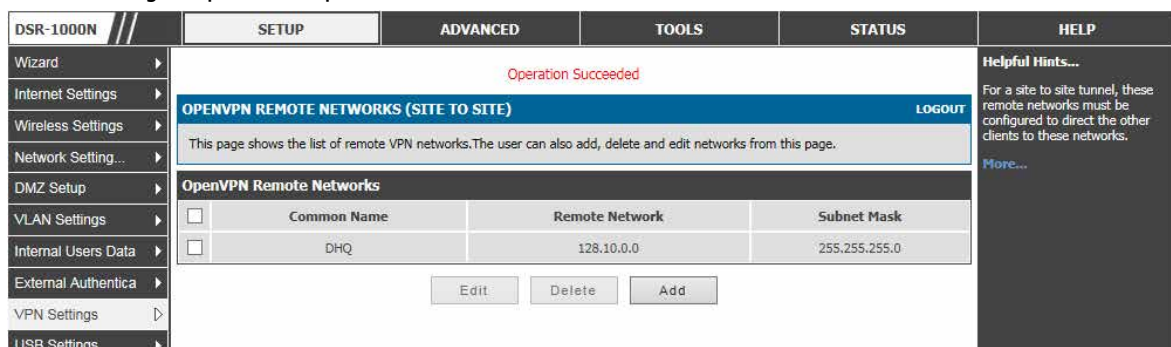
図 8-22 OpenVPN リモートネットワークリスト
