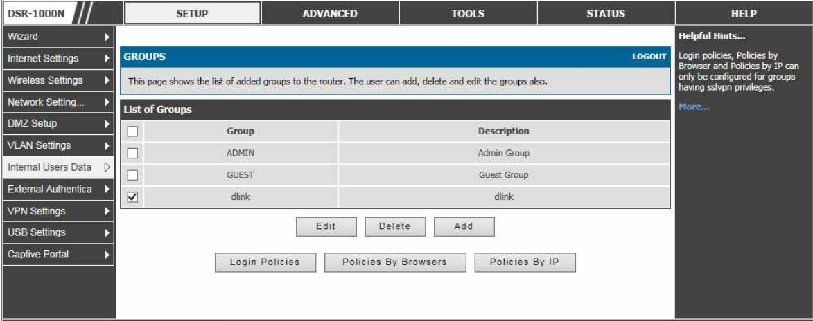
図 9-2 グループリスト
