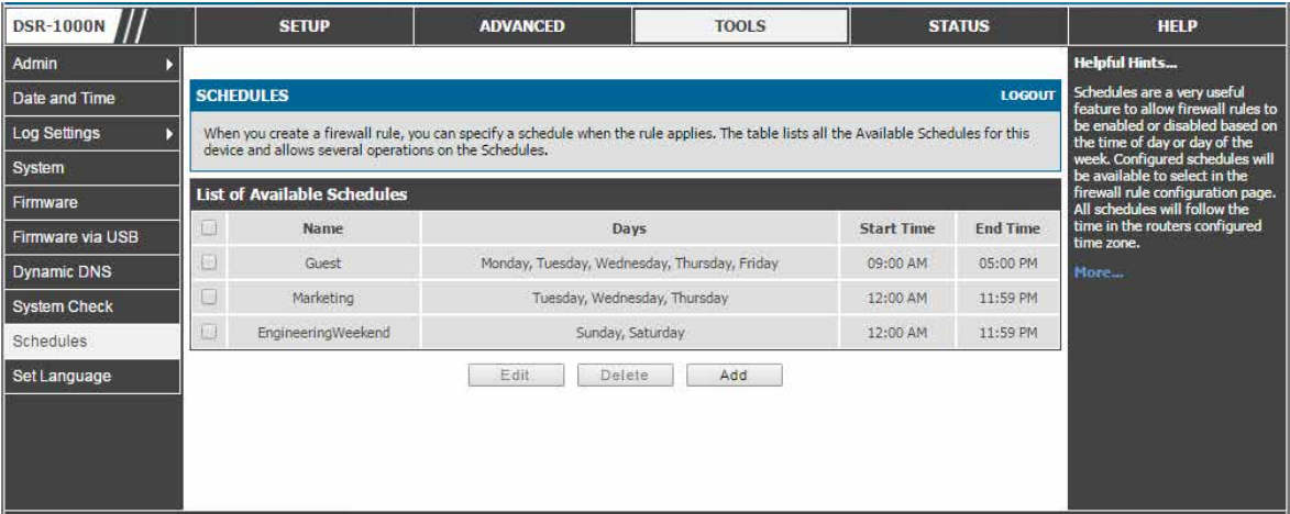
図 7-3 ファイアウォールにバインドする有効なスケジュールのリスト
