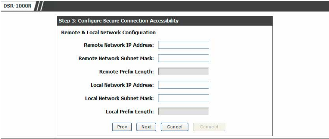
図 8-6 VPN ウィザード手順 3 画面
