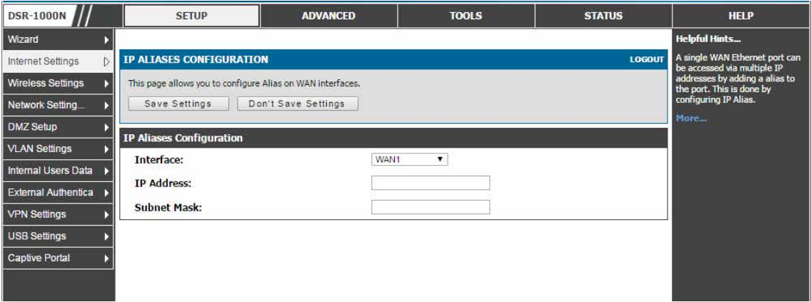
図 5-30 IP エイリアスの登録 画面
