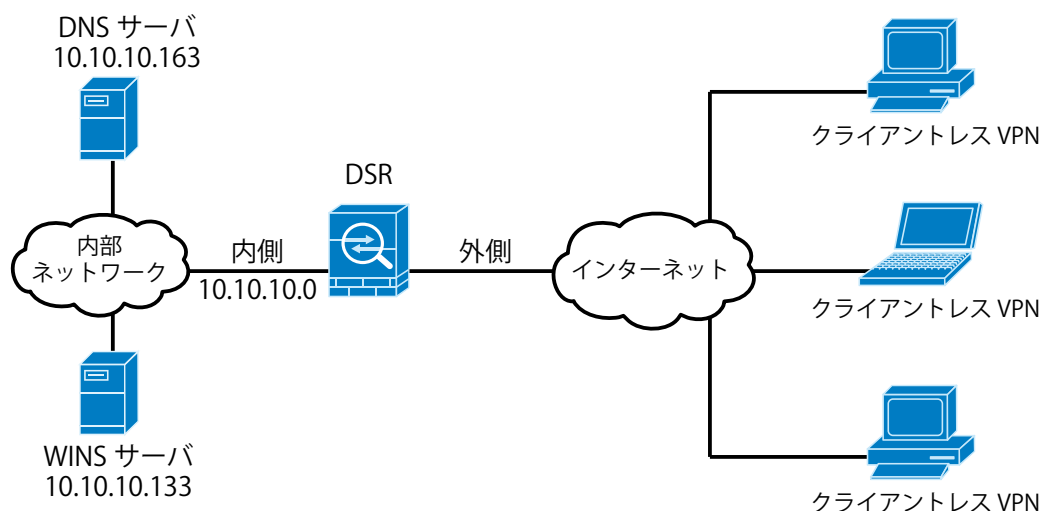
図 9-1 DSR へのクライアントレス SSL VPN 接続の例
