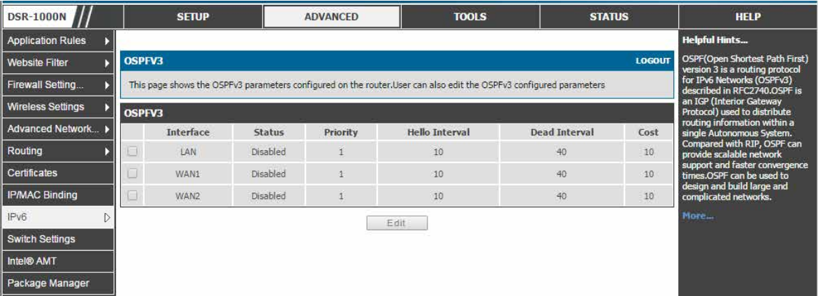
図 5-39 OSPFv3 の設定パラメータ
