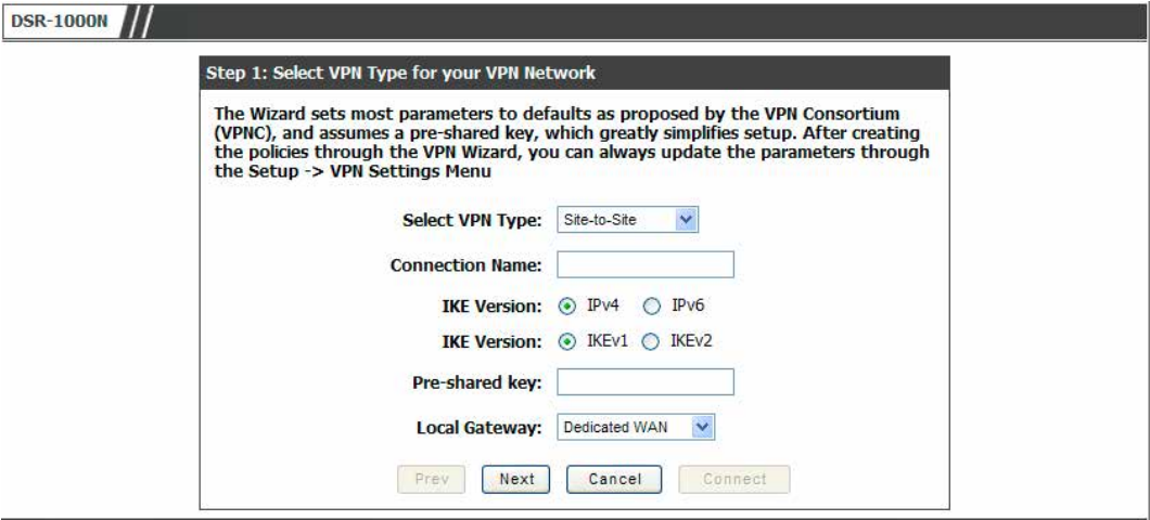
図 8-4 VPN ウィザード手順 1 画面
