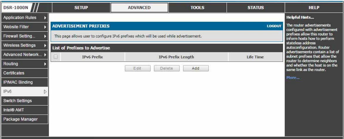
図 4-10 ADVERTISEMENT PREFIXES 画面
