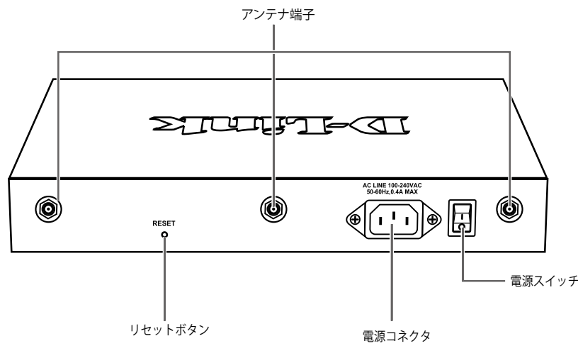
図 1-6 背面パネル図
