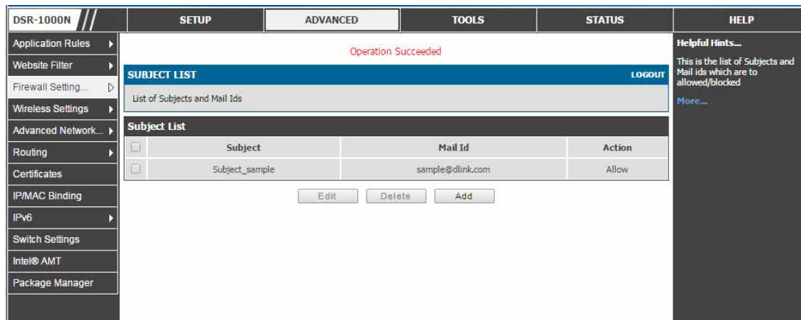
図 7-19 設定済みの題名
