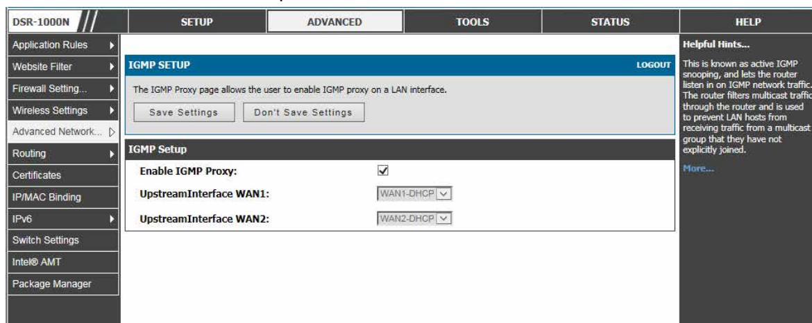
図 7-37 LAN への IGMP プロキシを有効にする
