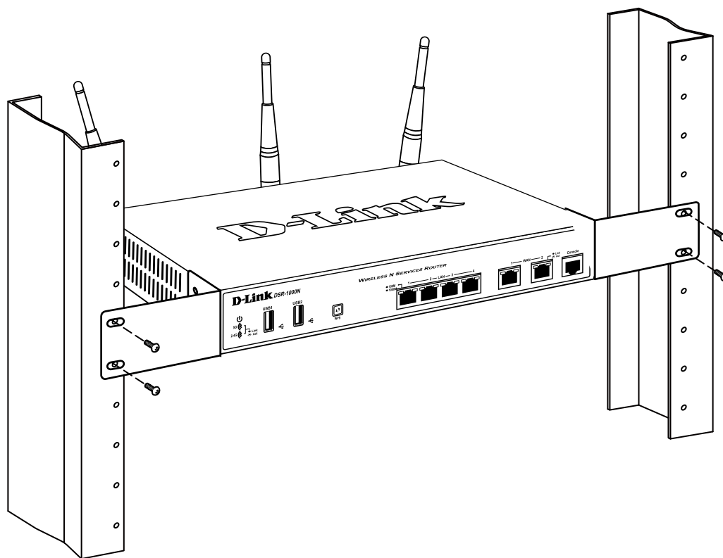
図 2-3 製品のラックへの設置
