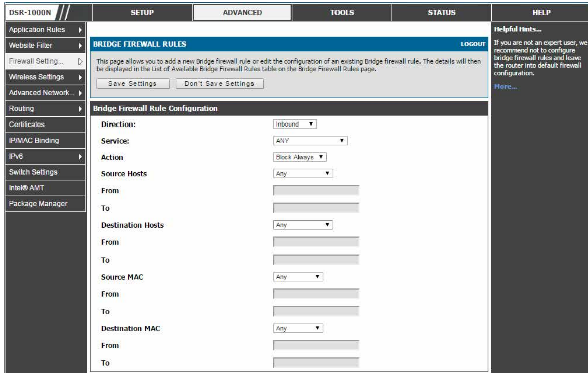
図 7-23 ブリッジファイアウォールルールの設定
