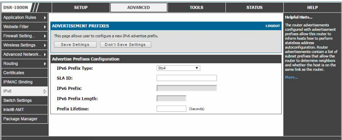
図 4-11 ADVERTISEMENT PREFIXES 画面 - 追加
