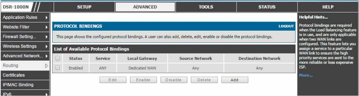
図 5-27 PROTOCOL BINDINGS 画面
