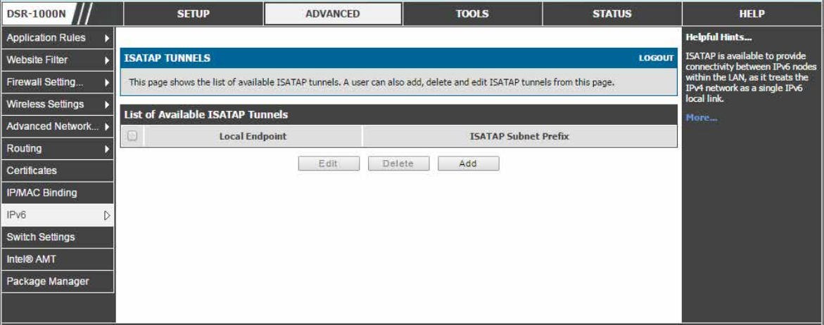
図 5-42 ISATAP トンネルのリスト
